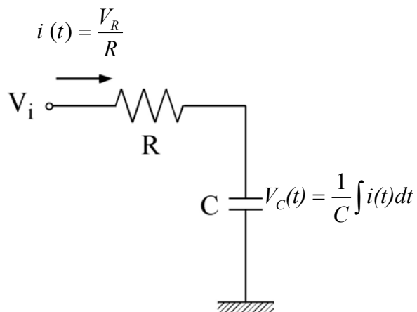
図 12-1 LPF 回路
