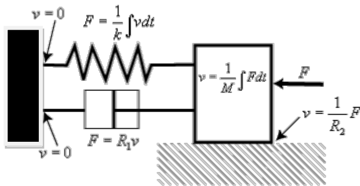
図 10-1 マス・ばね・ダンパーモデル
